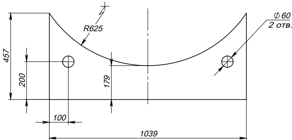
Поз.3 (Ребро)
