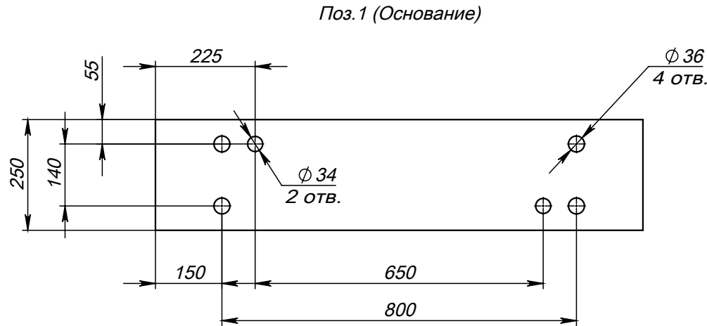
Поз.1 (Основание)
