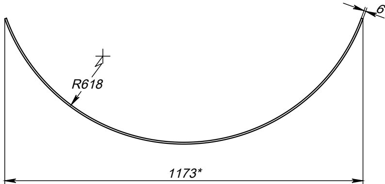
Поз.3 (Ребро)
